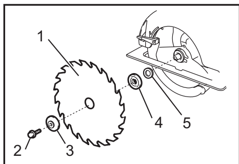
► 1. Disco de sierra 2. Tornillo hexagonal 3. Brida exterior 4. Brida interior 5. Anillo
